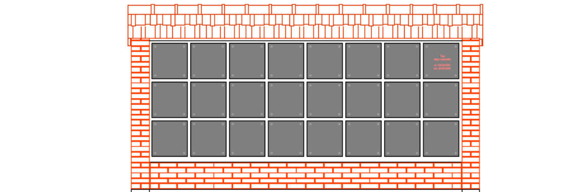
ELEWACJA FRONTOWA 1:25
